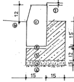
KRAWĘŻNIK NORMALNY
