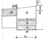
KRAWĘŻNIK TRAPEZOWY
