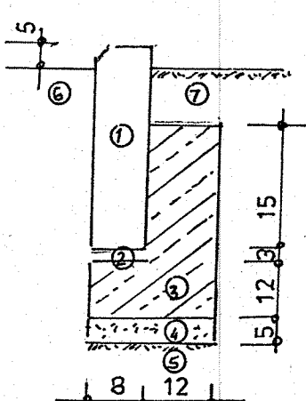
OBRZEŻE BETONOWE
