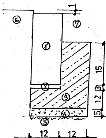
OPORNIK BETONOWY
