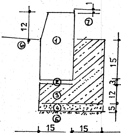
KRAWEŹNIK NORMALNY
