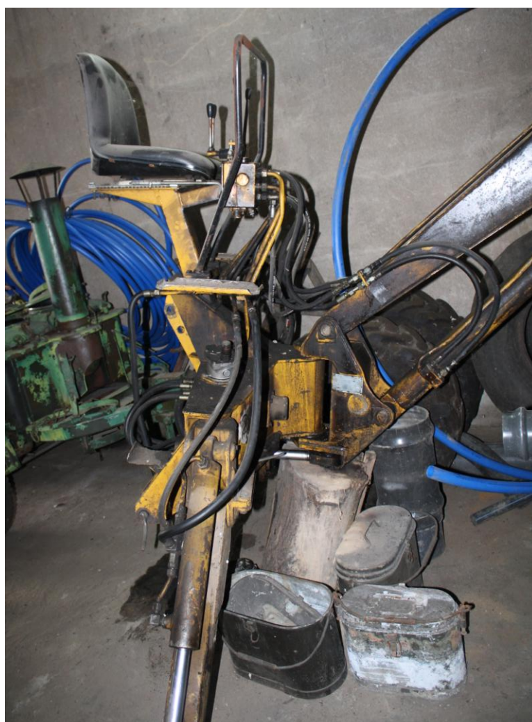
5. Koparko – ładowarka T-350/3 MIKRUS – 7.
